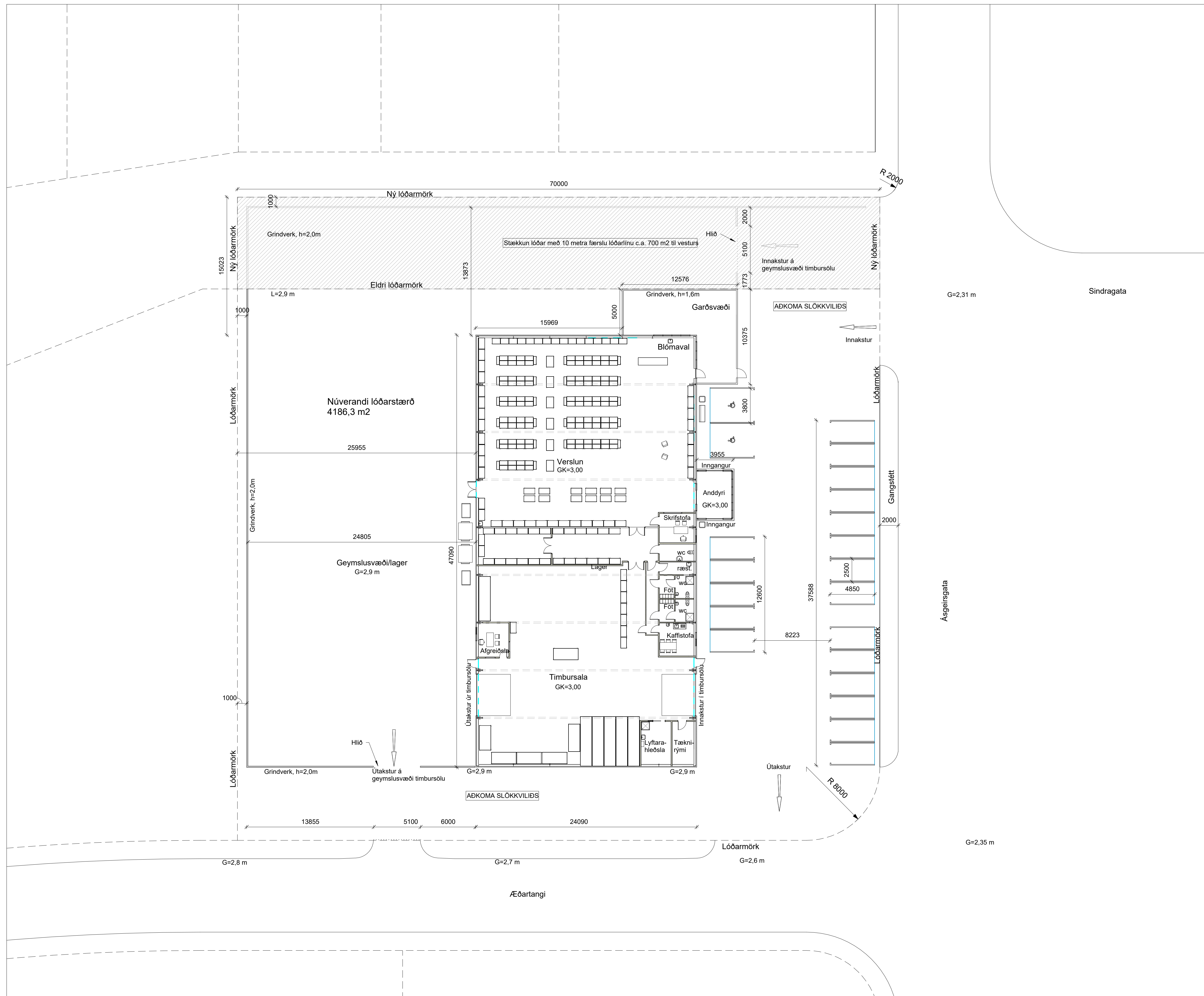
Lóðaruppráttur 1 : 200
