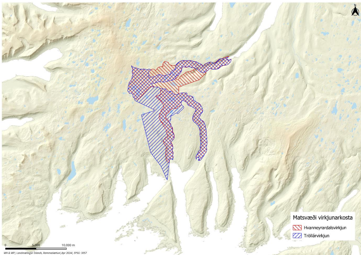
Mynd 7. Matsvæði fyrir Hvanneyrardalsvirkjun og Tröllárvirkjun skarast þar sem báðar byggjast á veitu vatns af fleiri en einu vatnasviði á einn stað til virkjunar, annars vegar niður í Ísafjörð og hins vegar niður í Vattarfjörð. Þessar virkjunarhugmyndir nýta því að hluta til sama vatnið (krossstrikað svæði á korti) og útiloka þar með hvor aðra.
