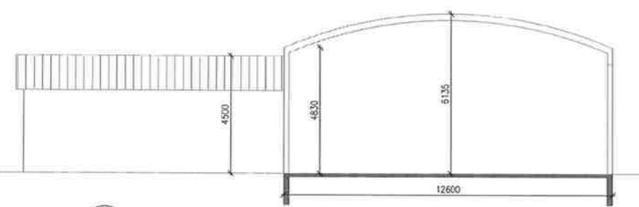
D Snið C40.001 1:100
