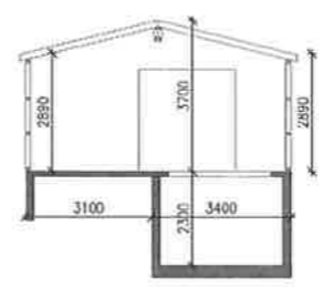
A Snið C40.001 1:100
