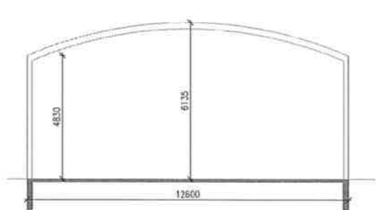
C Snið C40.001 1:100
