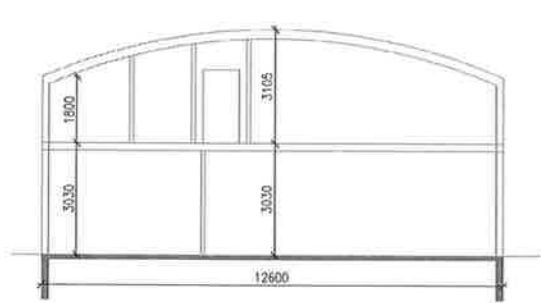
B Snið C40.001 1:100
