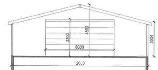
E Snið C40.001 1:100
