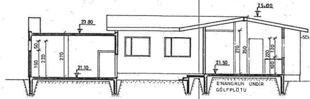
SKURÐUR A-A
