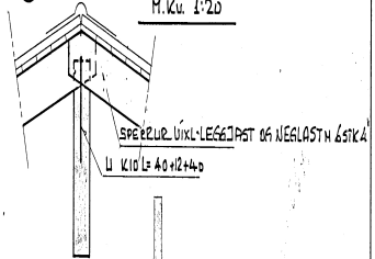
2 SNID Í SPERUR Á MIEM M.KV. 1:20
