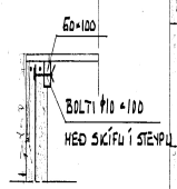
4. SNID Í GÖFLS PERUR M.KV. 1:20
