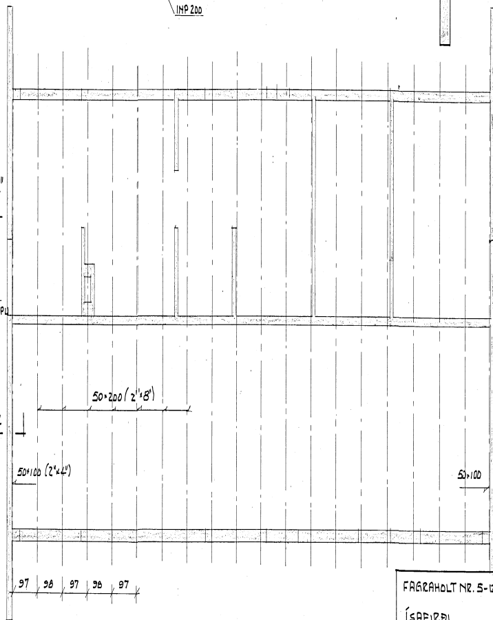
4. SNID Í GÖFLS PERUR M.KV. 1:20
