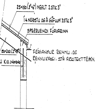
2 SNID Í SPERUR Á MIEM M.KV. 1:20
