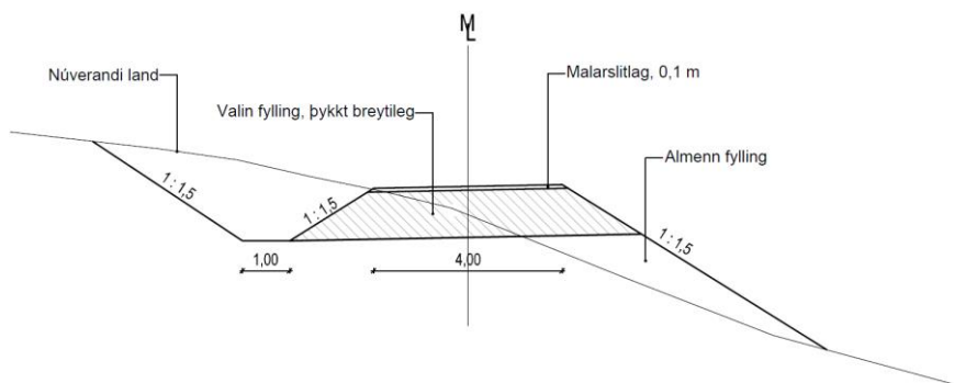
Mynd 3.12 Dæmigert þversnið vinnuvegar (Verkís).
