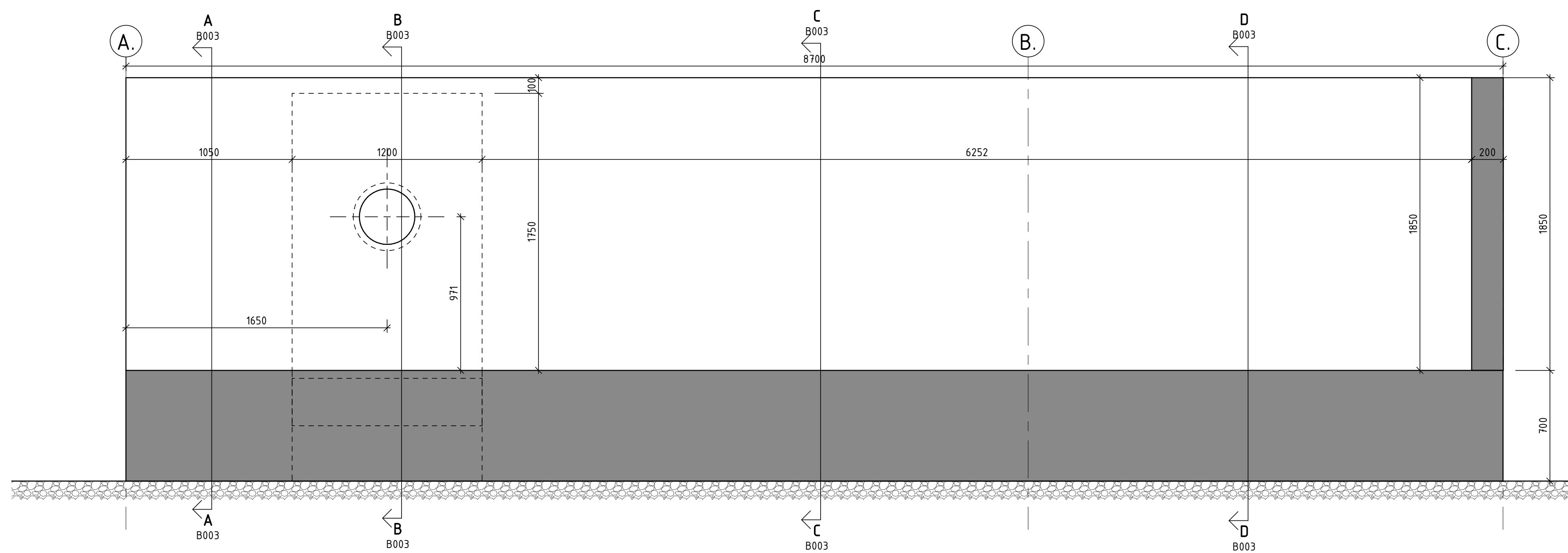
SNID G-G, FORM 1 : 20
