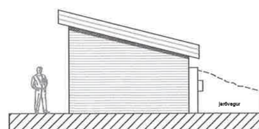
ÚTLIT HLIÐ 1:100
