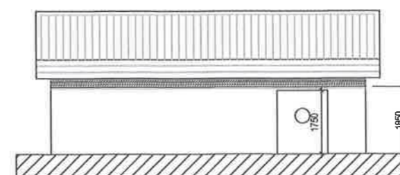
ÚTLIT AFTAN 1:100
