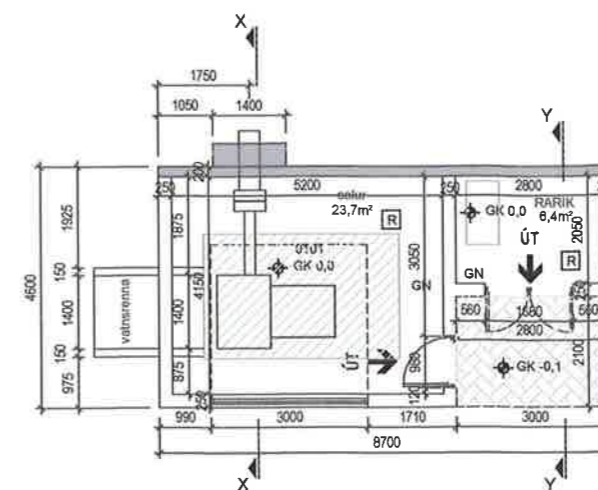
GRUNNMYND 1:100
