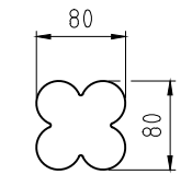
Stolpe skala 1:5
