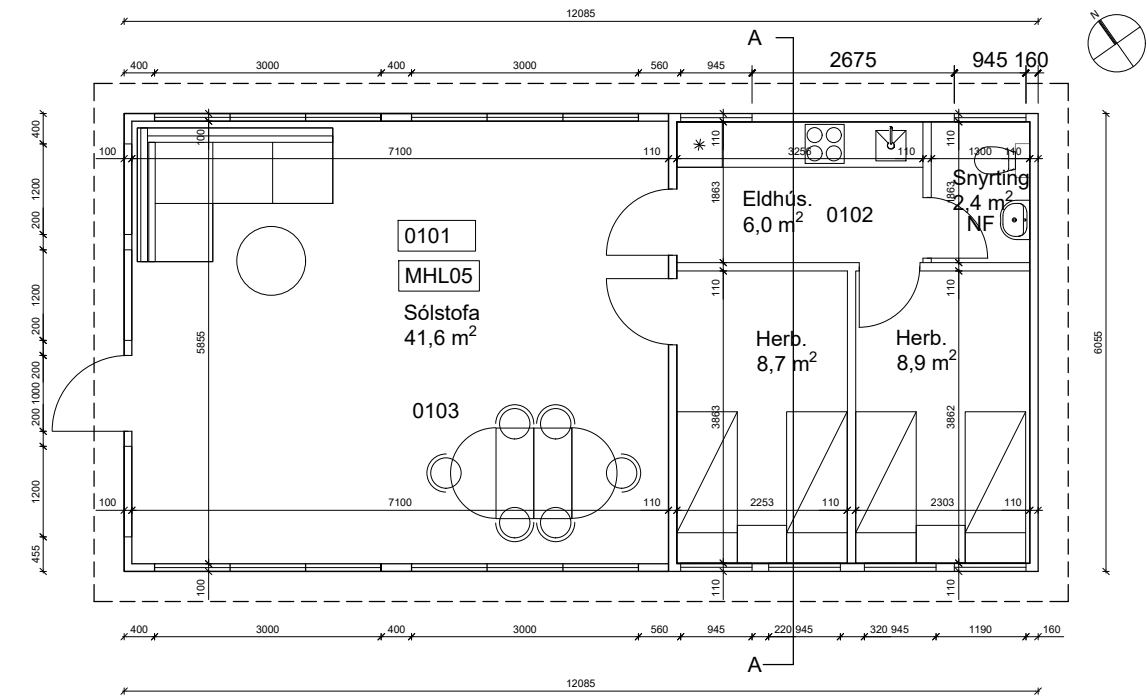
Grunnmynd 1.hæð mkv. 1:100
