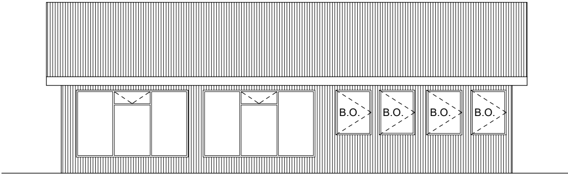
Útlit suð-vestur- mkv. 1:100
