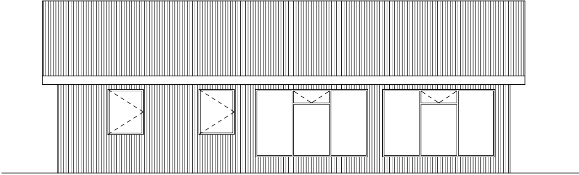
Útlit norð-austur- mkv. 1:100
