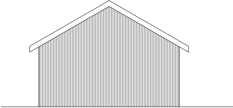
Útlit suð-austur - mkv. 1:100
