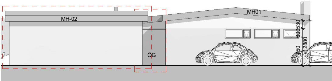
Útlit - Norðaustur 1:100
