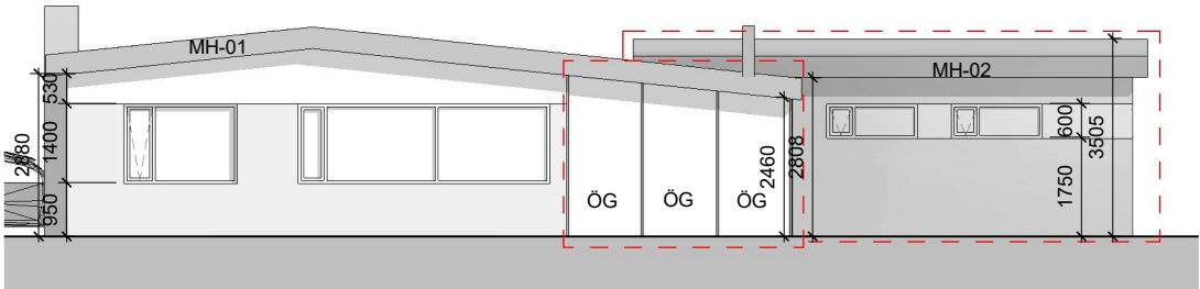
Útlit - Suðvestur 1:100
