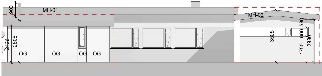
Útlit - Suðaustur 1:100
