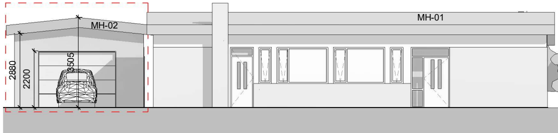
Útlit - Norðvestur 1:100
