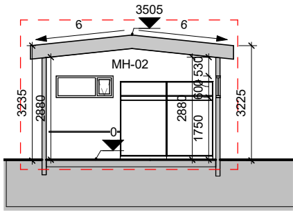
Snið 2 - Bílgeymsla 1:100
