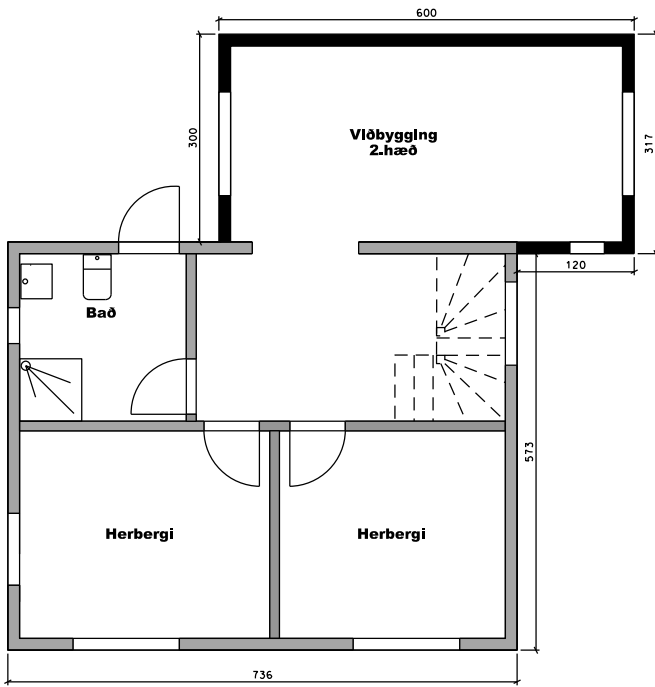
Grunnmynd 2. hæð
