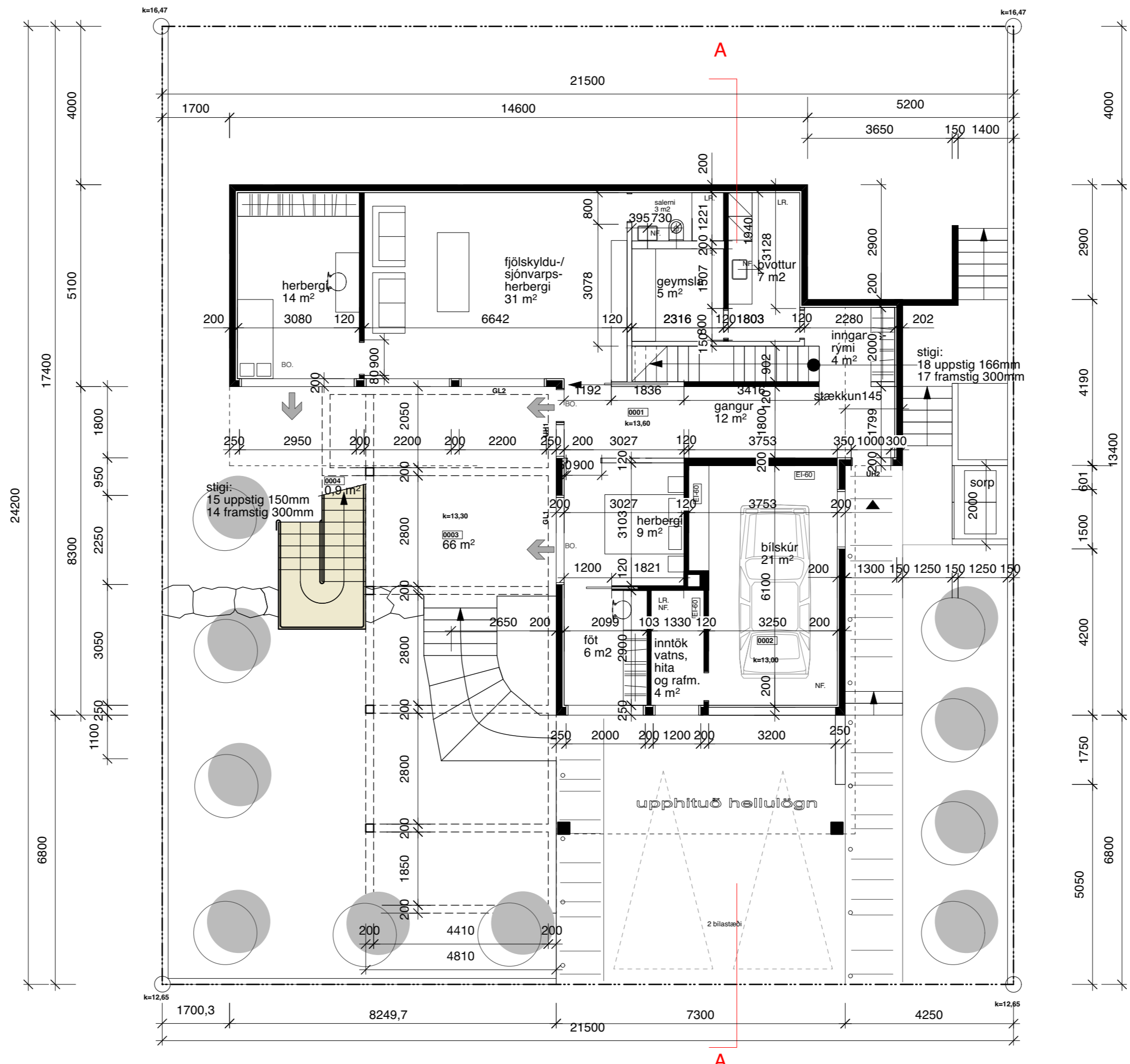
KJALLARI m.kv. 1:100
