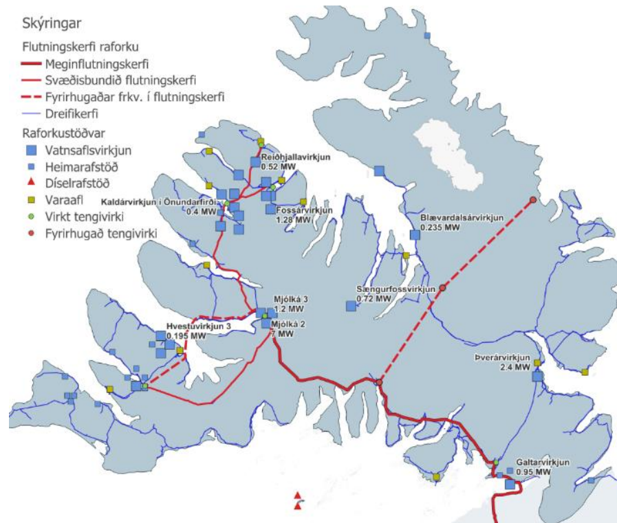
Mynd 4-10 Raforkuframléiðsla, flutningskerfi og dreifikerfi raforku.
