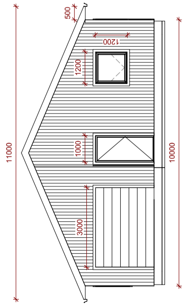
3 VESTUR 1 : 100
