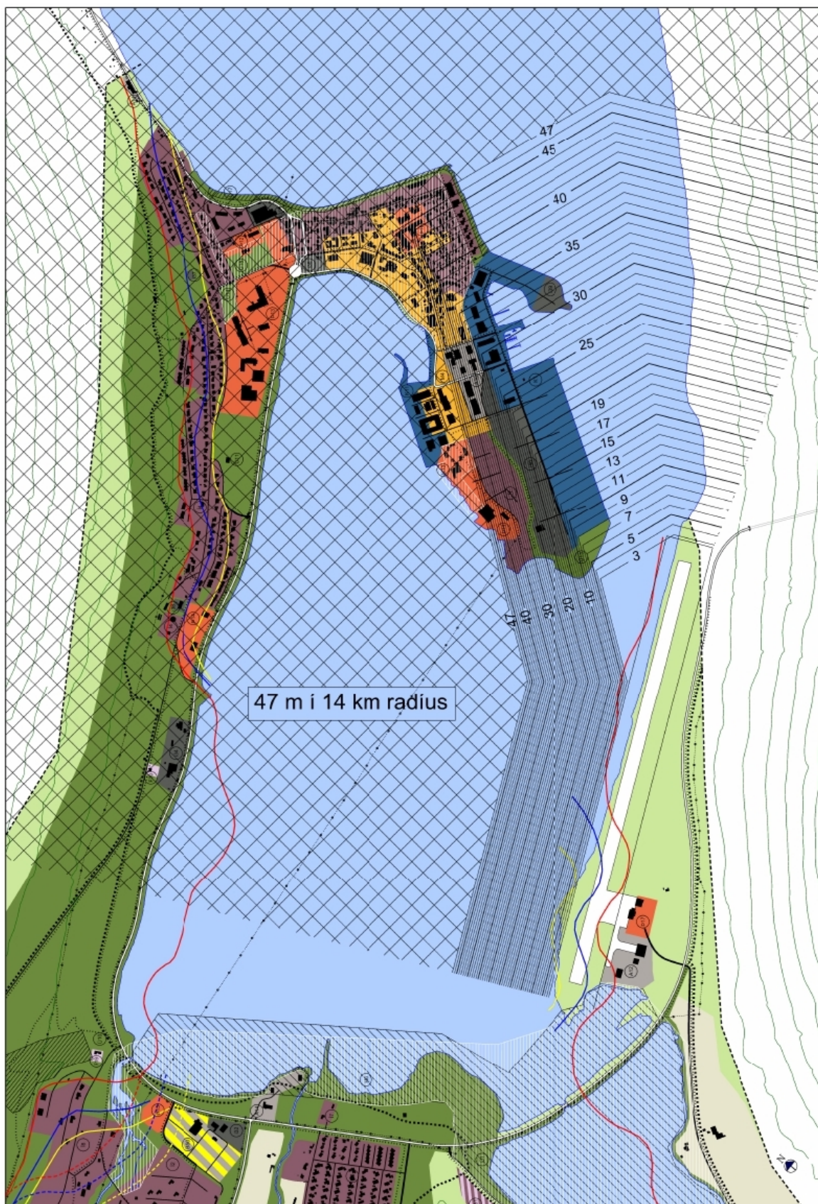
Mynd 12.1. Hindranaflötur Ísafjarðarflugvallar.
