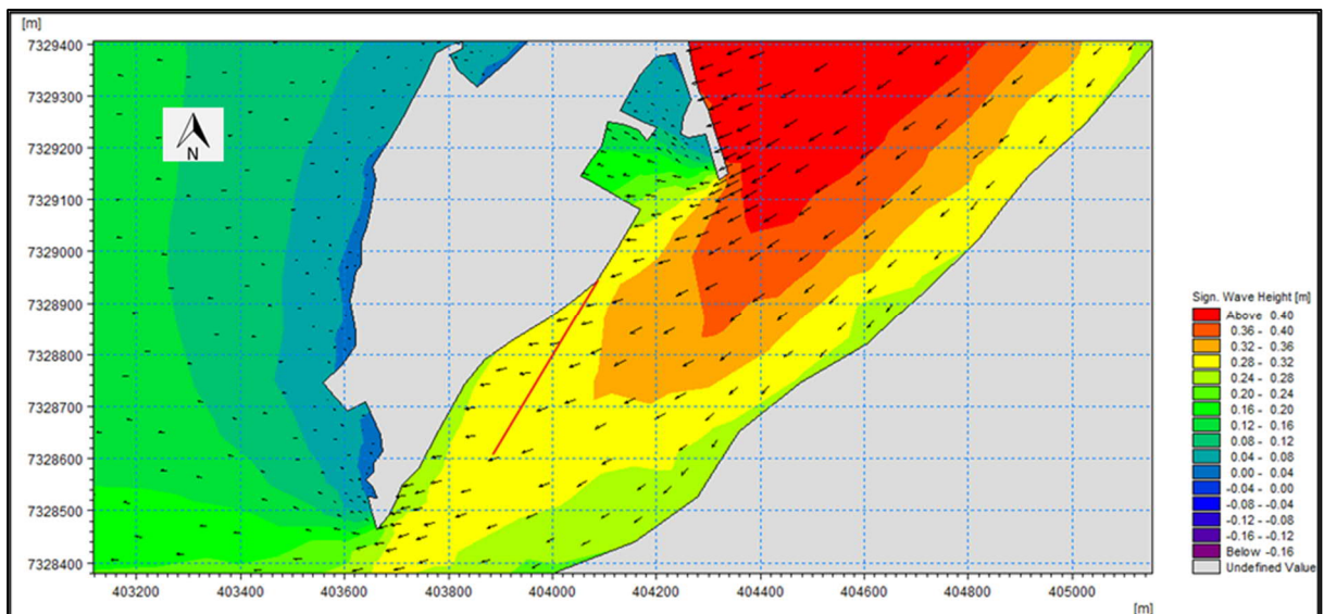
Mynd 6.6 Kennialda og öldustefna 98% austan vindöldu. Lenging Sundabakka hefur verið teiknuð með rauðri línu. Hér táknar guli liturinn 0,28 – 0,32m ölduhæð. 33
