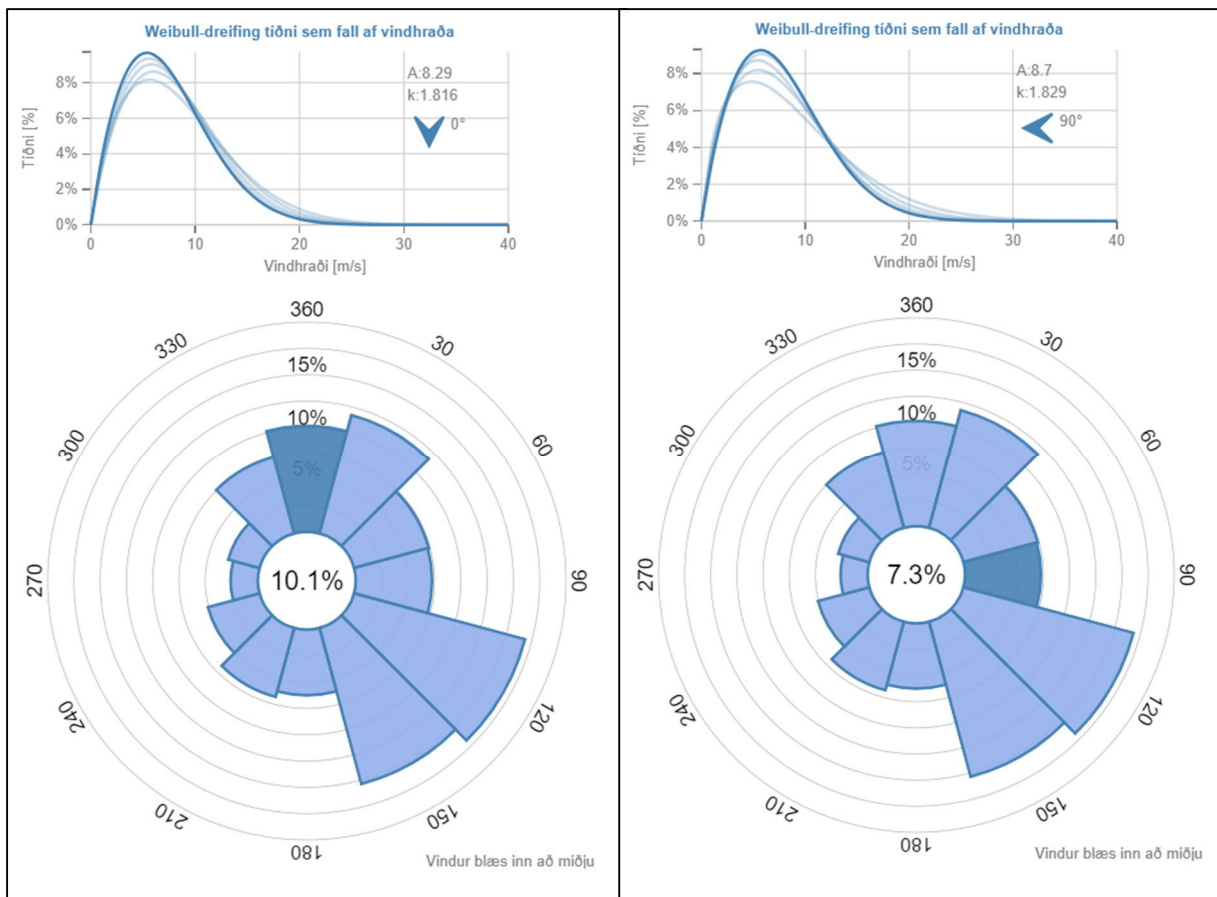
Mynd 6.4 Vindrós við mynni skutulsfjarðar og dreifingu vindhraða úr norðri (vinstri) og austri (hægri). 33
