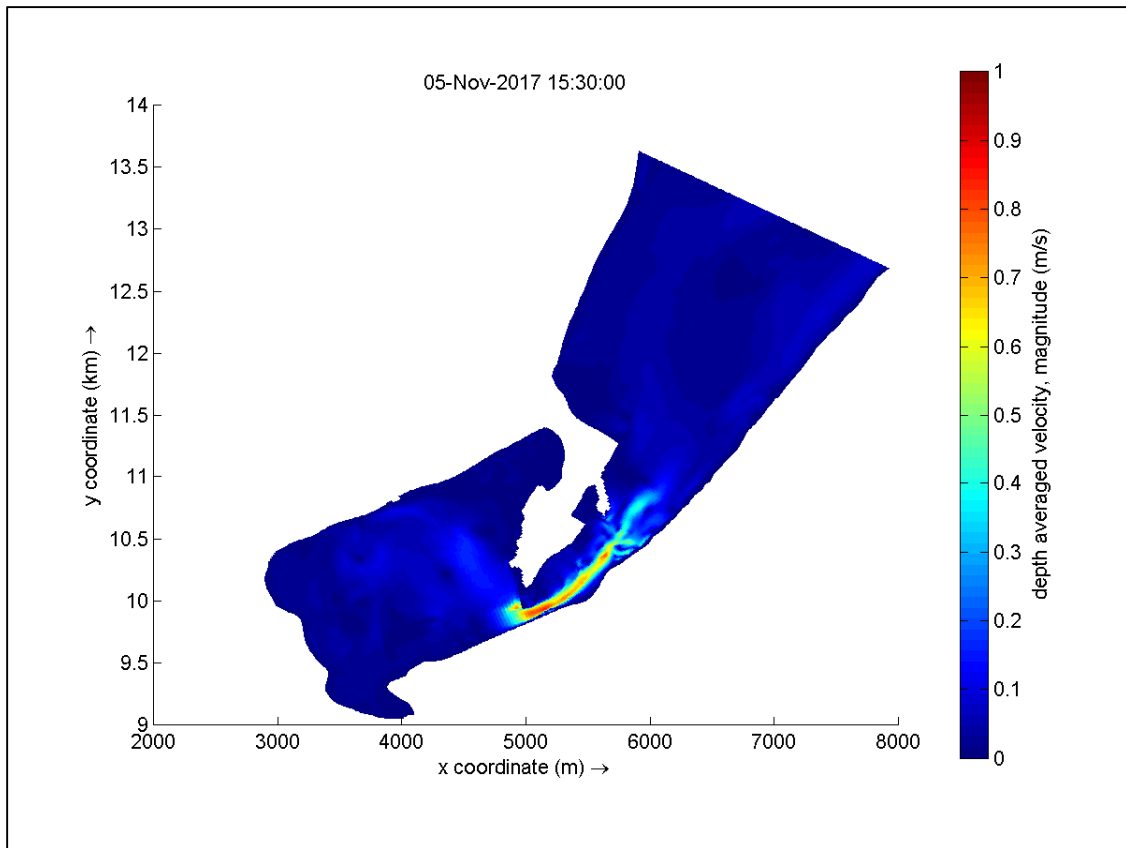
Mynd 6.2 Straumhraði á svæðinu nálægt stórstraumsfjöru þegar útfall er í hámarki. 31
